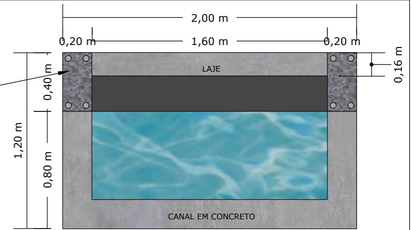
Detalhamento Canal Esc. 1:25
