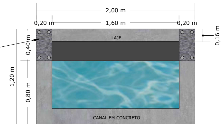
Detalhamento Canal Esc. 1:25
